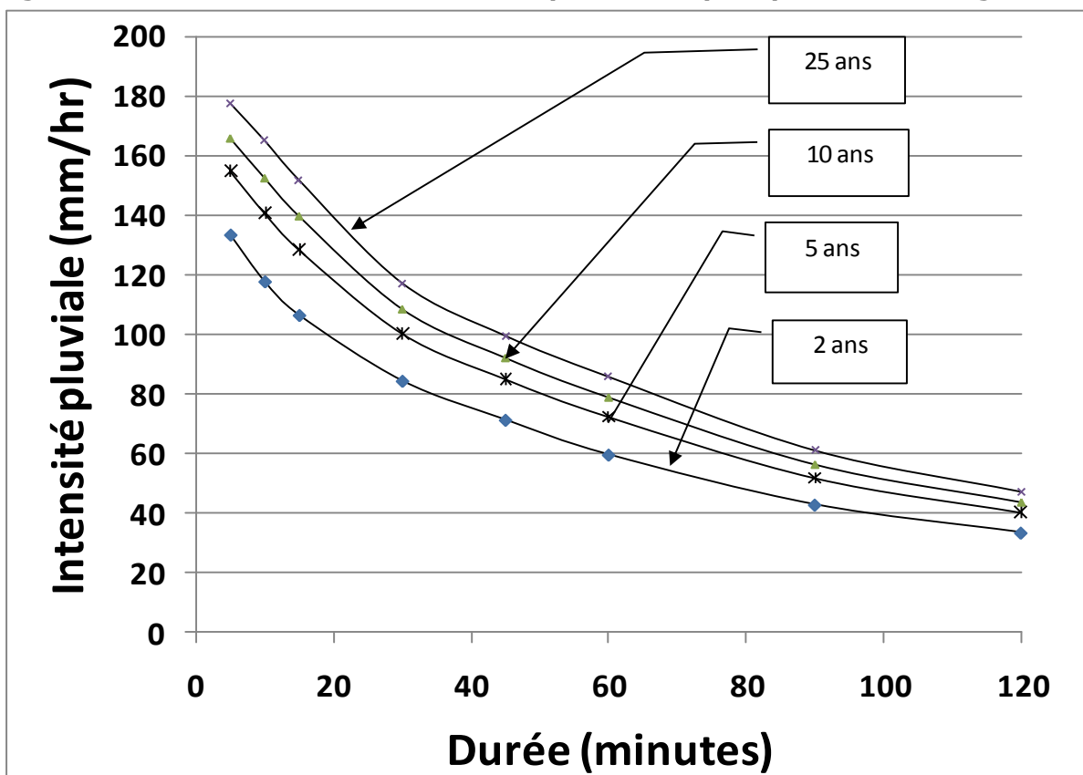
Figure 2-9 Courbes Intensité-Durée-Fréquence des précipitations à Bangui
